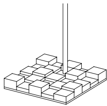
BBAS/L1 dim. 40x40xSP6 cm basamento in legno massiccio wooden dice base
